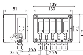
Beépítési méretek DCU YPV SCI 1000 2M
