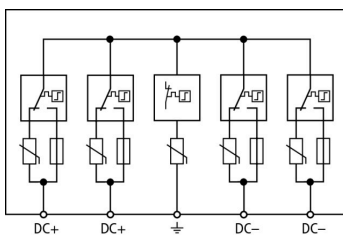
Kapcsolási rajz DCU YPV SCI 1000 2M
